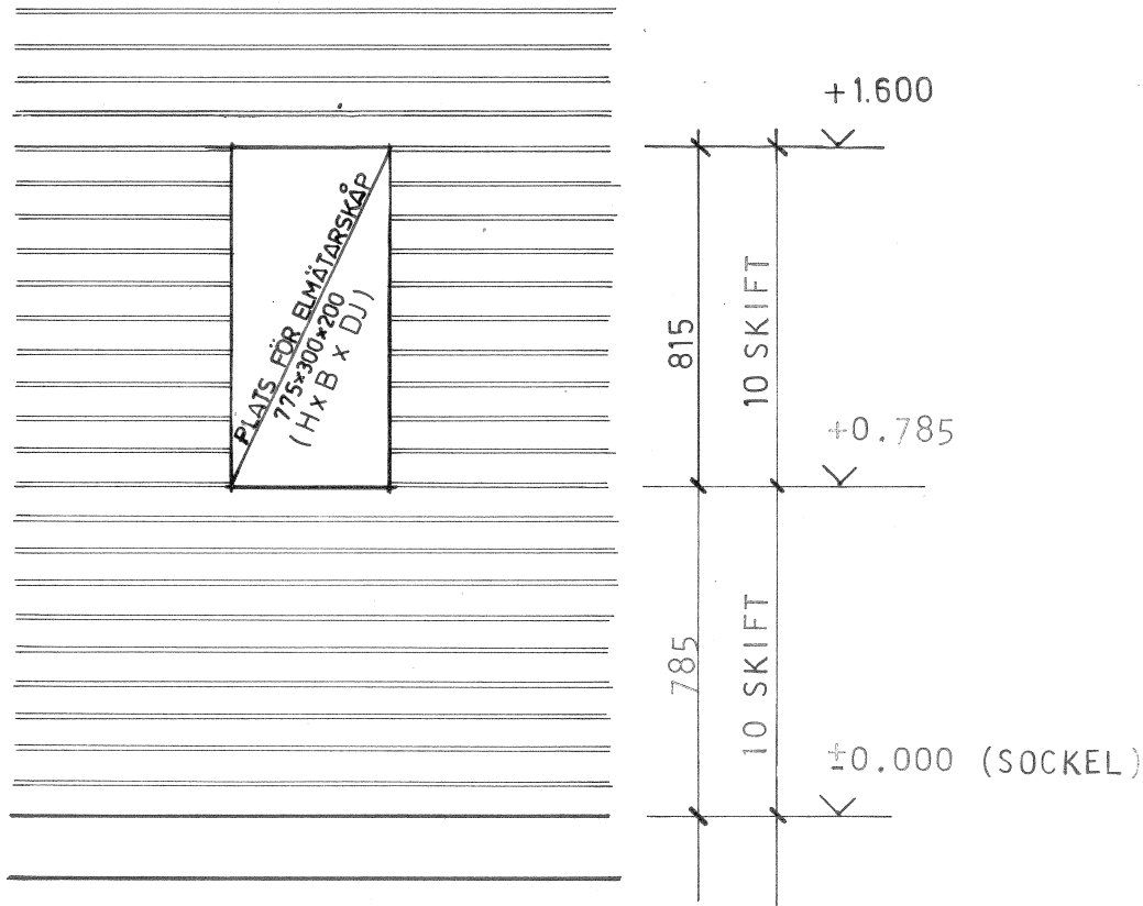
FASAD
